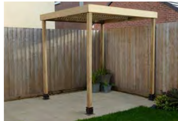
MODULAR PERGOLA – NO SIDES MODPERG(HD) 205(h) x 197(w) x 197(d)cm
