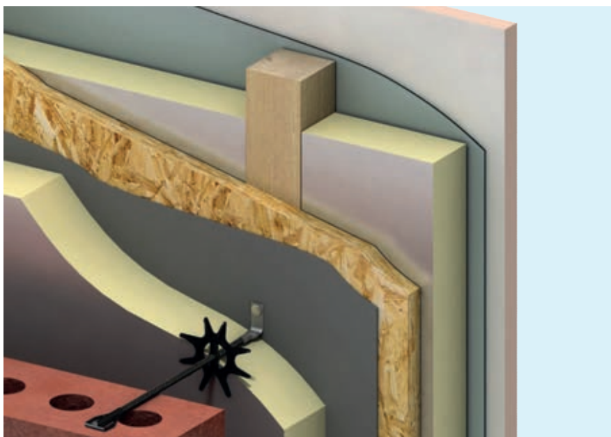
Ancon Teplo-BFL-Tie (Type 6)
