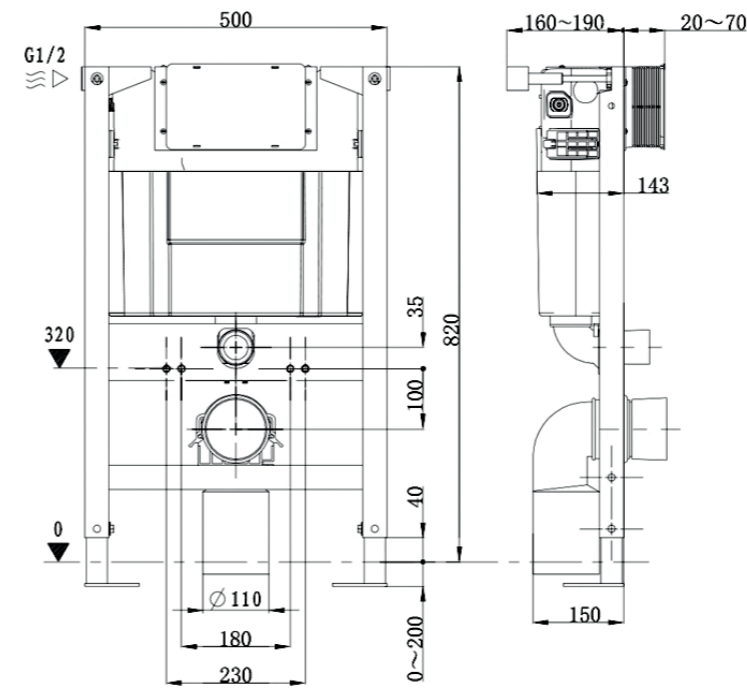
MODFR820 | 820mm
