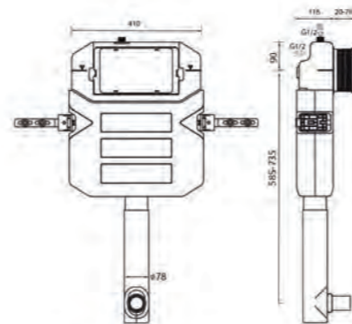
MODCIST1180 | 1180mm
