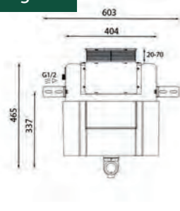
MODCIST820 | 820mm
